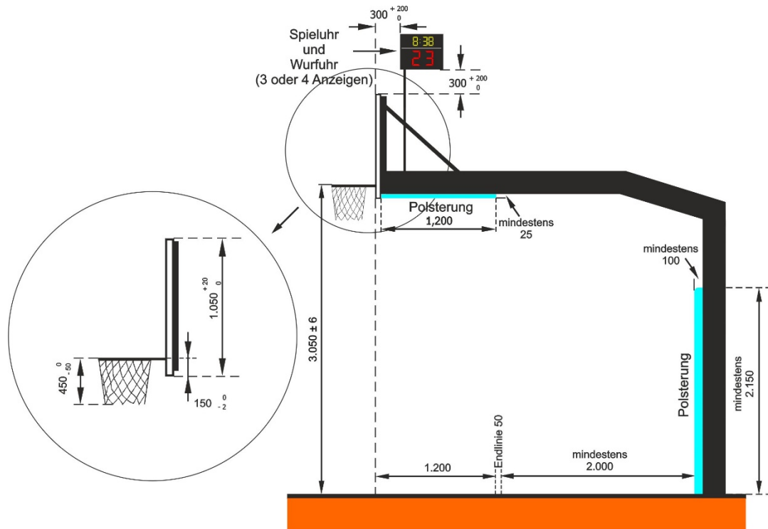
Bild 1 Korbanlage Stufe 1 (Wurfuhr Option 1)
