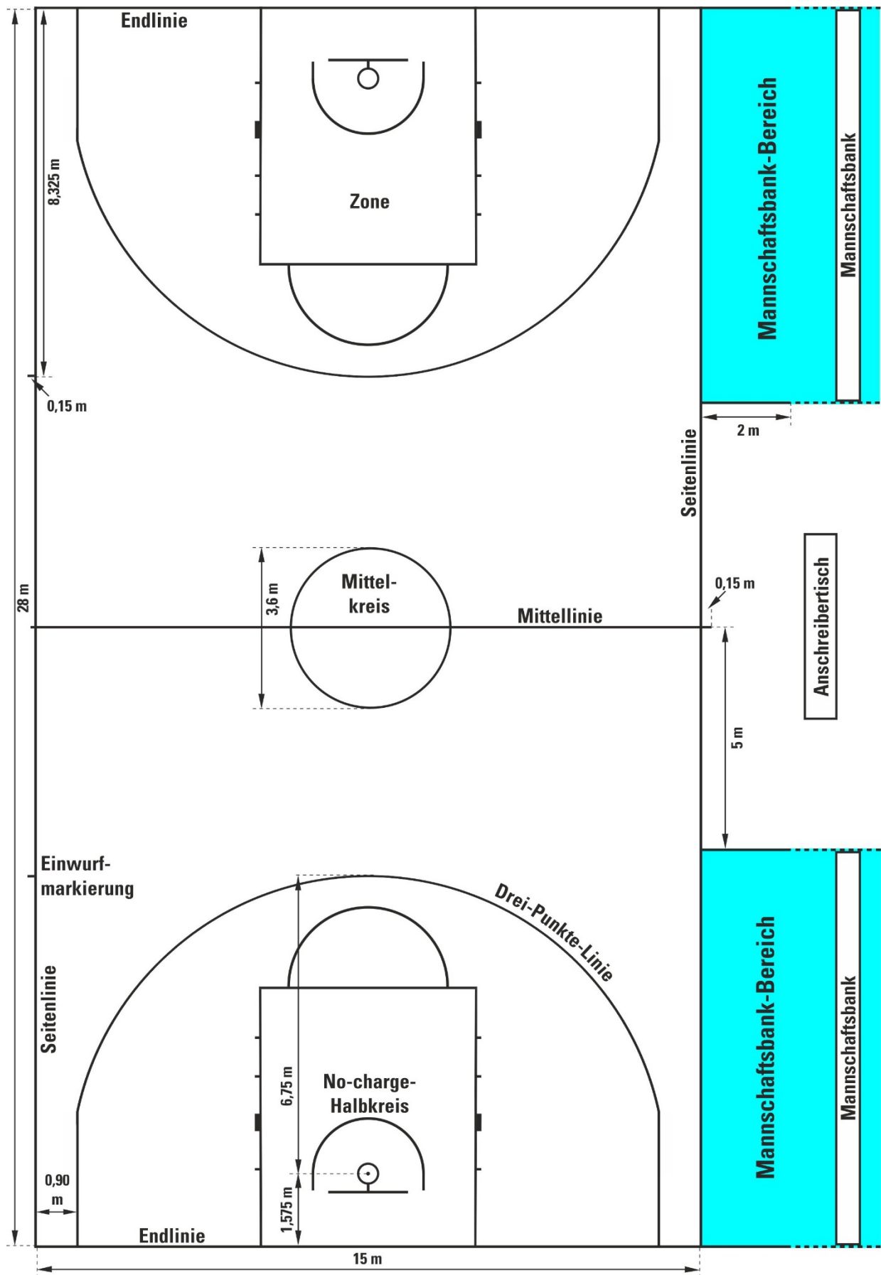
Bild 1 Vorschriftsmäßiges Spielfeld
