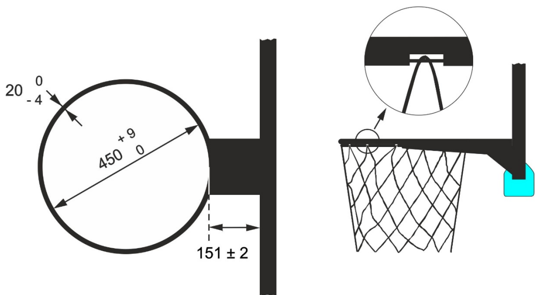
Bild 4 Ringabmessungen
