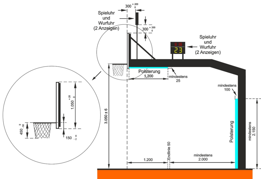
Bild 2 Korbanlage Stufe 1 (Wurfuhr Option 2)
