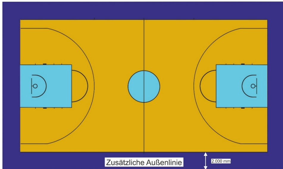
Bild 12 Spielfeld
